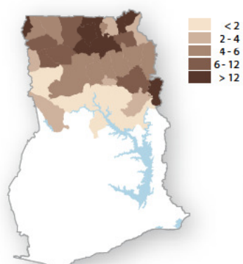
Millet
