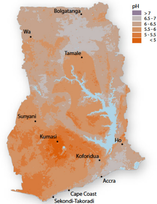
pH
